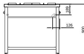
CONEXÃO DE GÁS 1/2" NPT VISTA LATERAL
