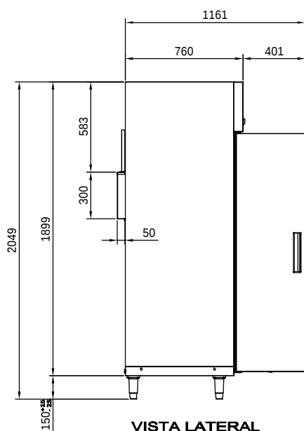
VISTA LATERAL
