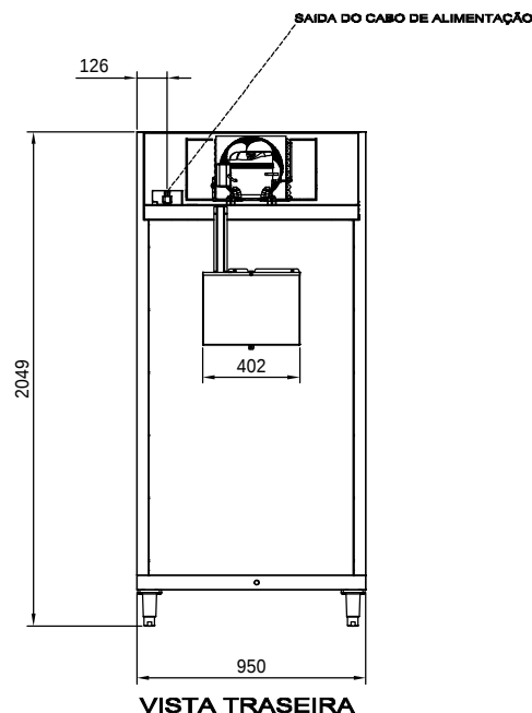
VISTA TRASEIRA
